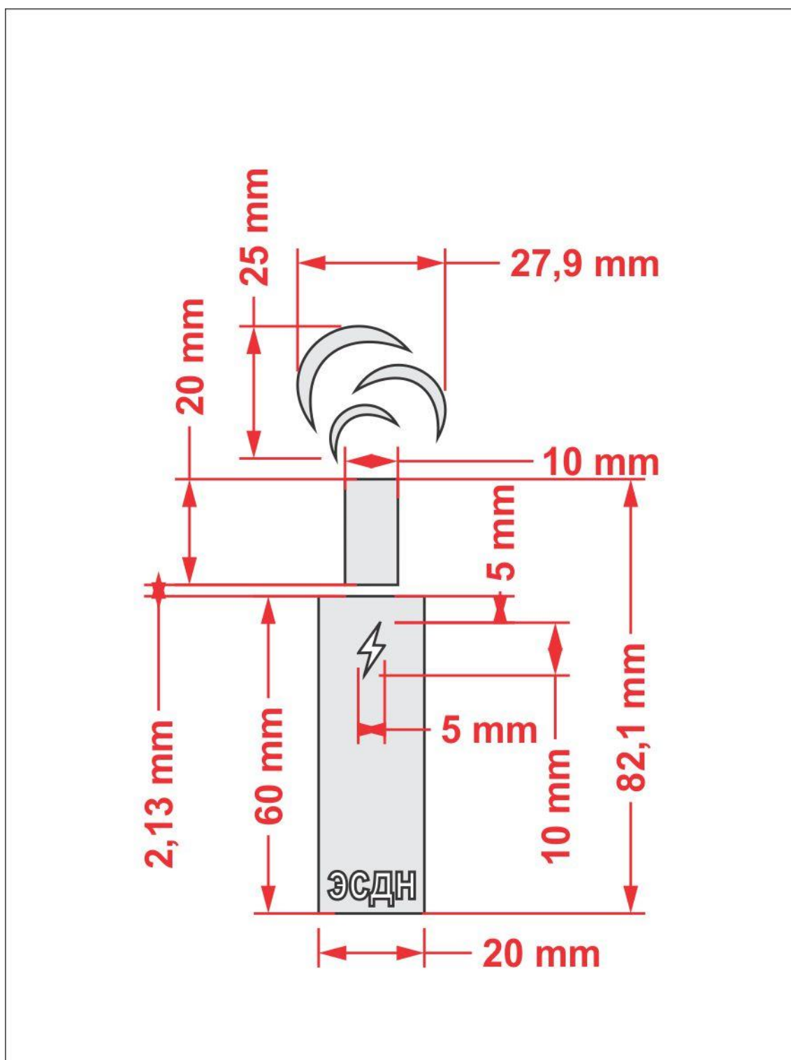
Схема расположения и размеры составляющих графического символа (элемента) «электронная сигарета» (ЭСДН)
