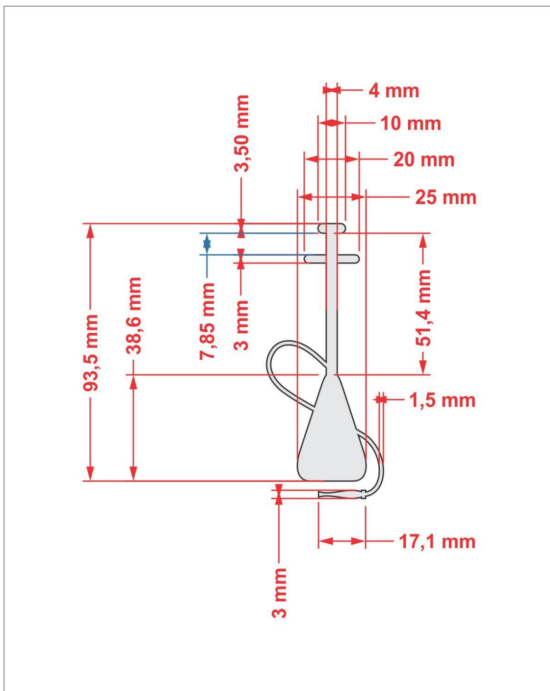
Схема расположения и размеры составляющих графического символа (элемента) «кальян»
